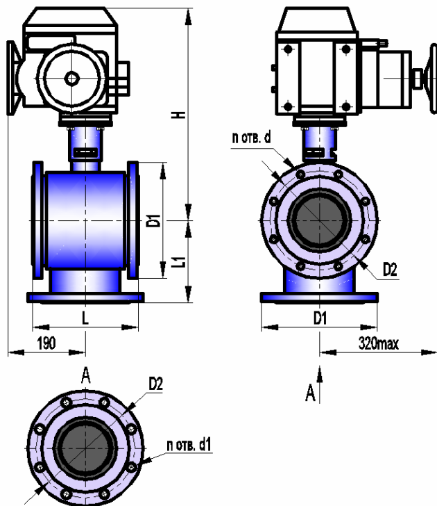
Габаритно-присоединительные размеры, мм
