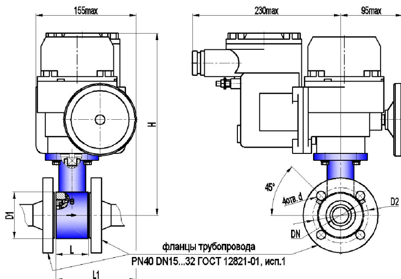
Габаритно-присоединительные размеры, мм
