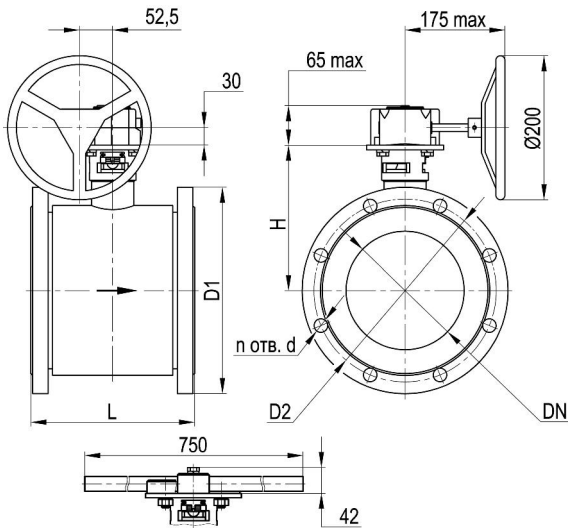
Габаритно-присоединительные размеры, мм
