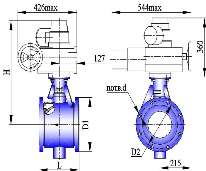
Габаритно-присоединительные размеры, мм
