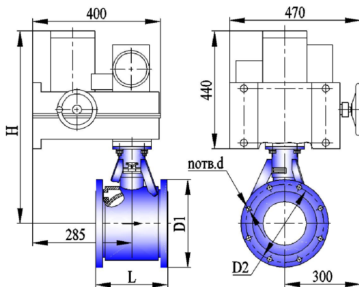
Габаритно-присоединительные размеры, мм
