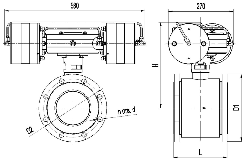
Габаритно-присоединительные размеры, мм
