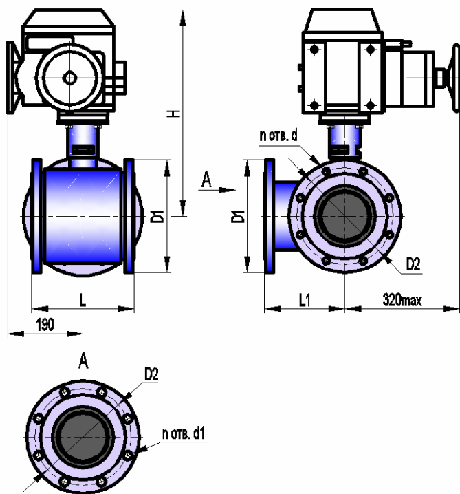
Габаритно-присоединительные размеры, мм
