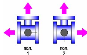
Схема переключения потока
