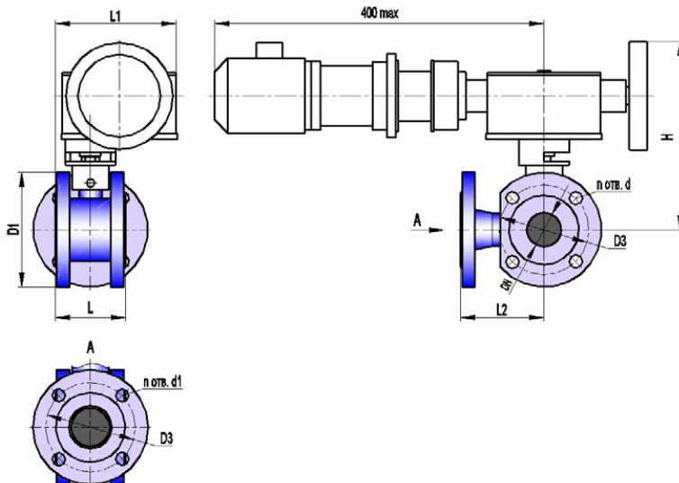
Габаритно-присоединительные размеры, мм
